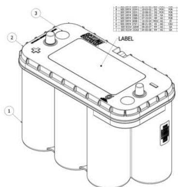
Disegno tecnico
