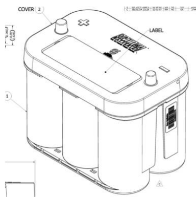
Disegno tecnico
